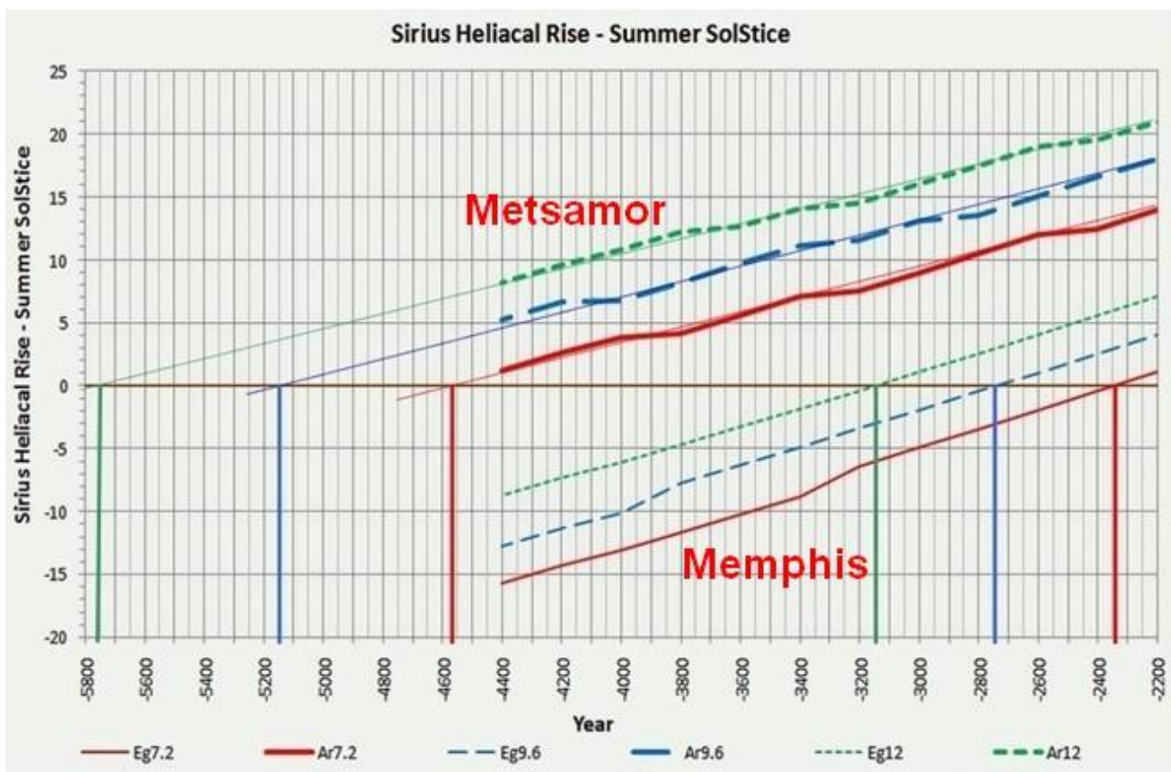
Рис.2 Расчет совпадения дней гелиакического восхода Сириуса и дня летнего солнцестояния для различных углов погружения Солнца для Мецамора (Ar7.2, Ar9.6, Ar12) и Мемфиса (Eg7.2, Eg9.6, Eg12).
